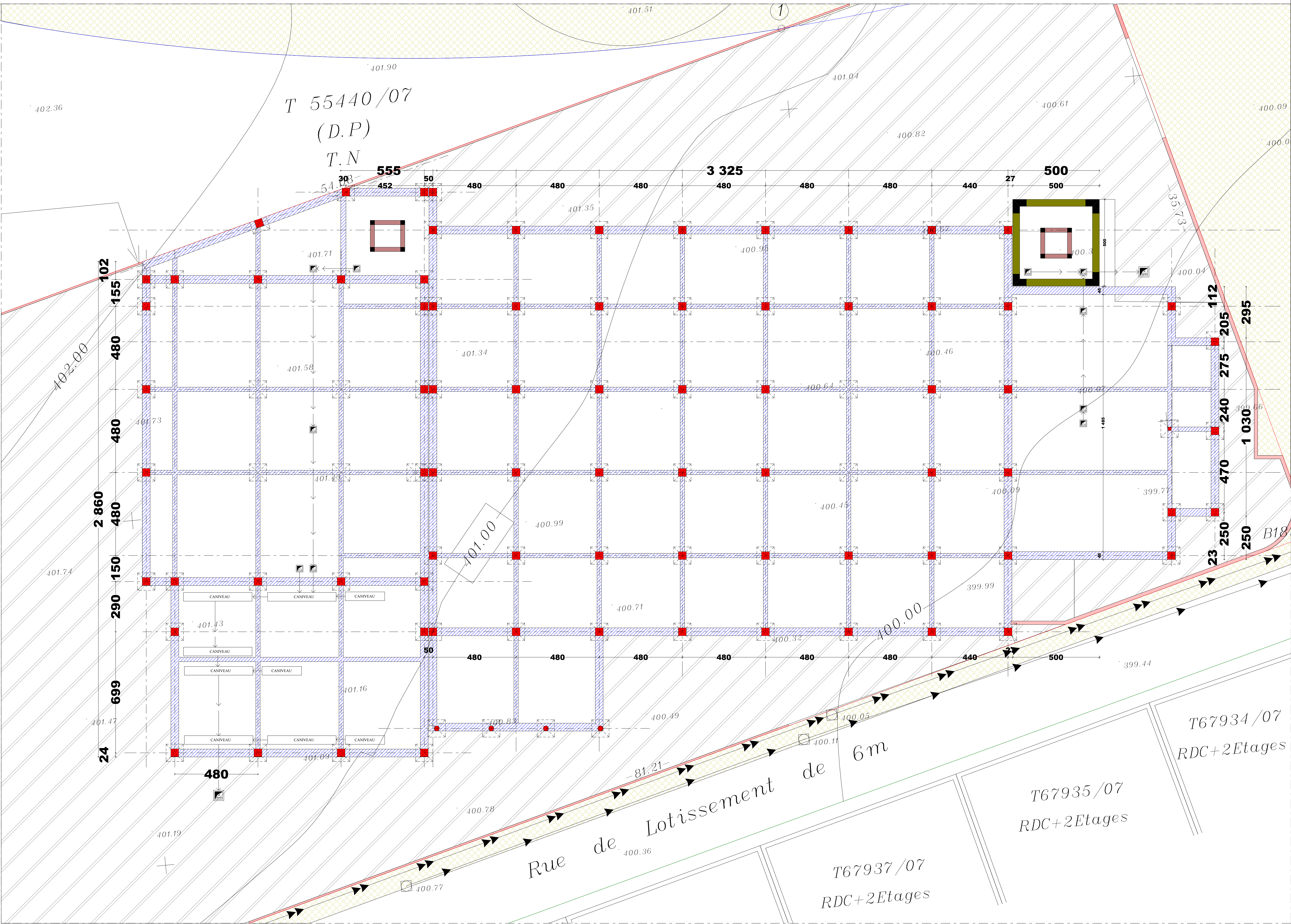
PLAN FONDATION
