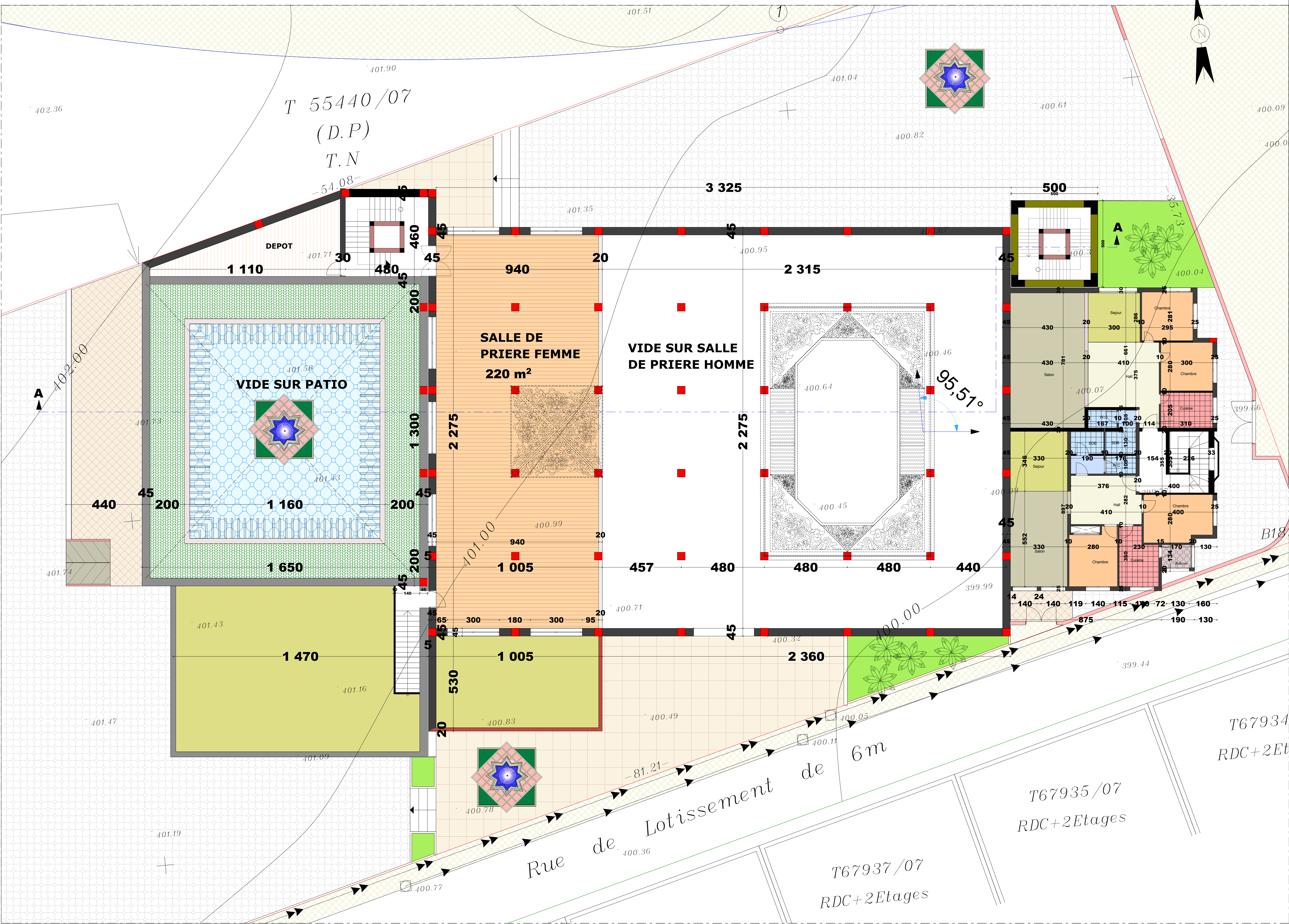
PLAN ETAGE
