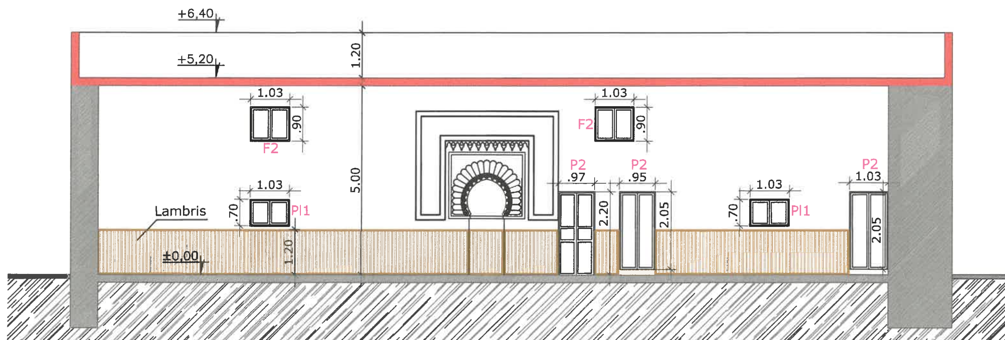
Etat Projeté
