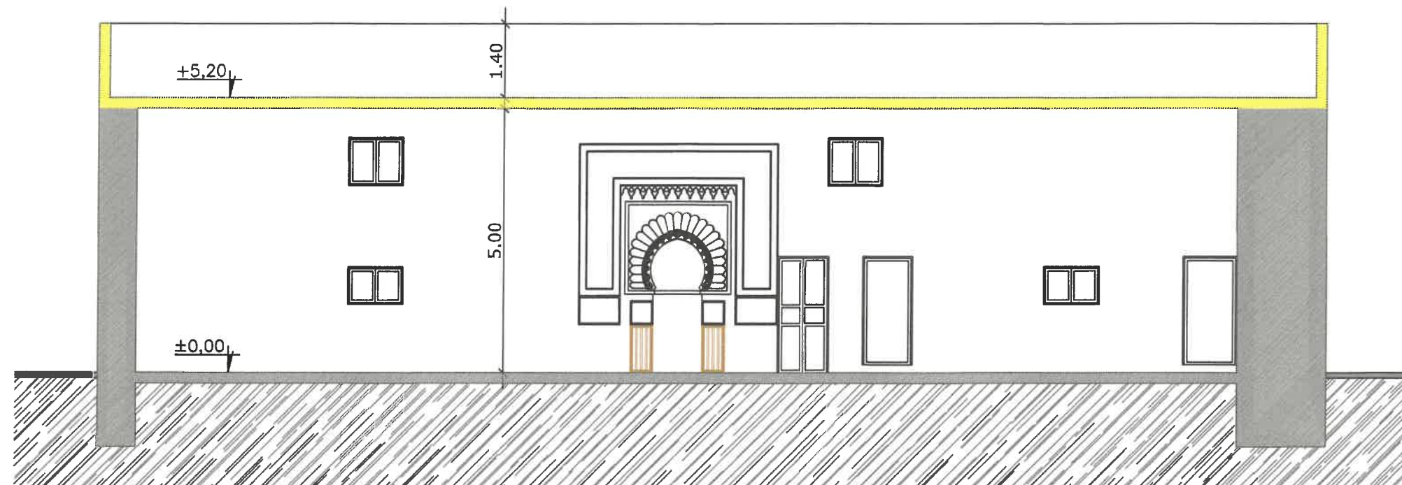
Etat Existant
