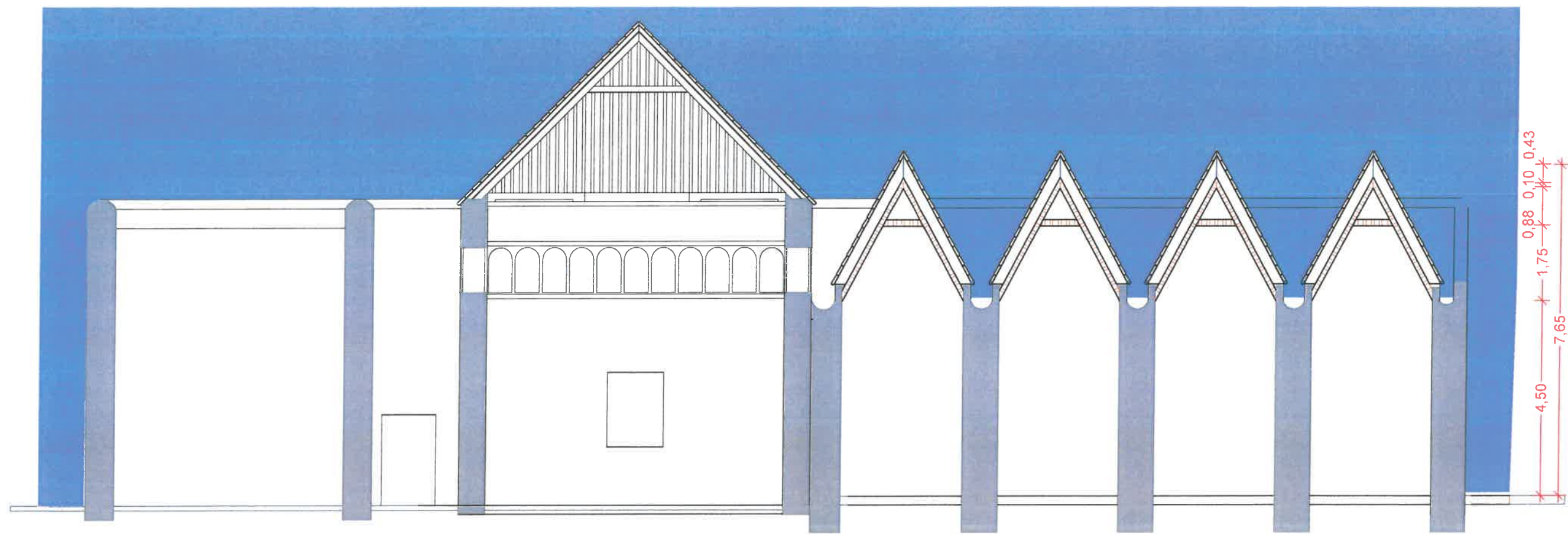
Coupe C C Proposition Apres Restauration
