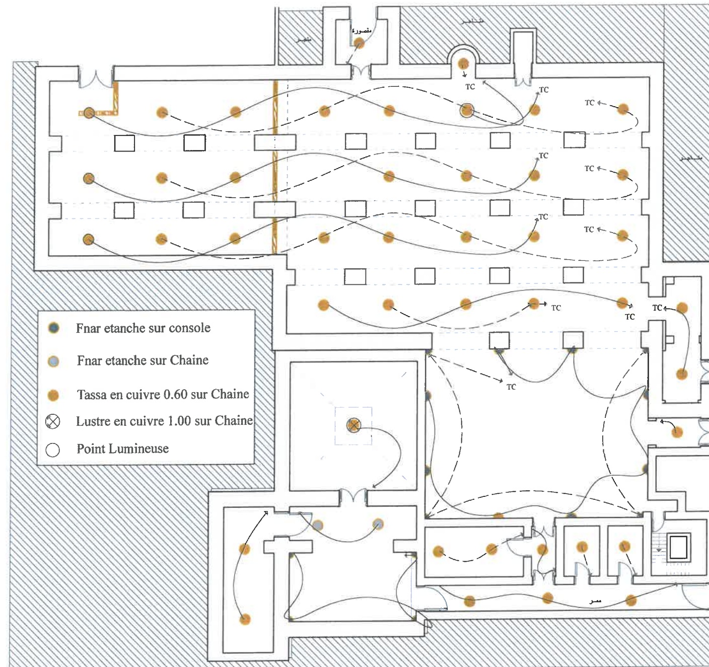
RDC REPERAGE ELECTIQUE
