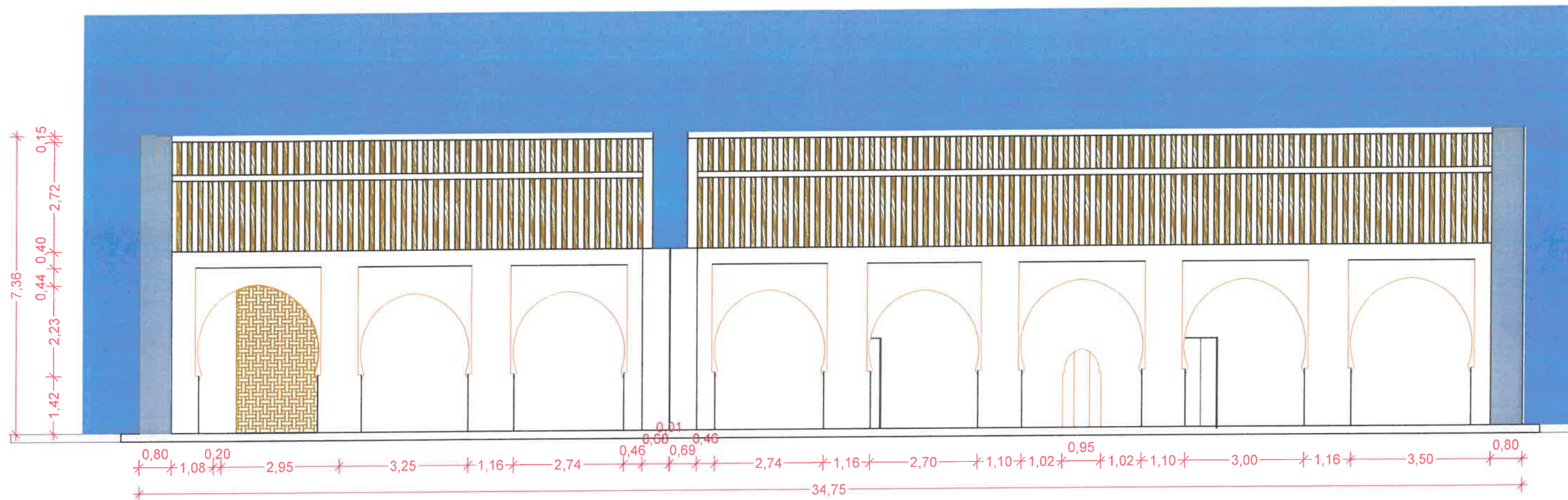
Coupe A A Proposition Apres Restauration
