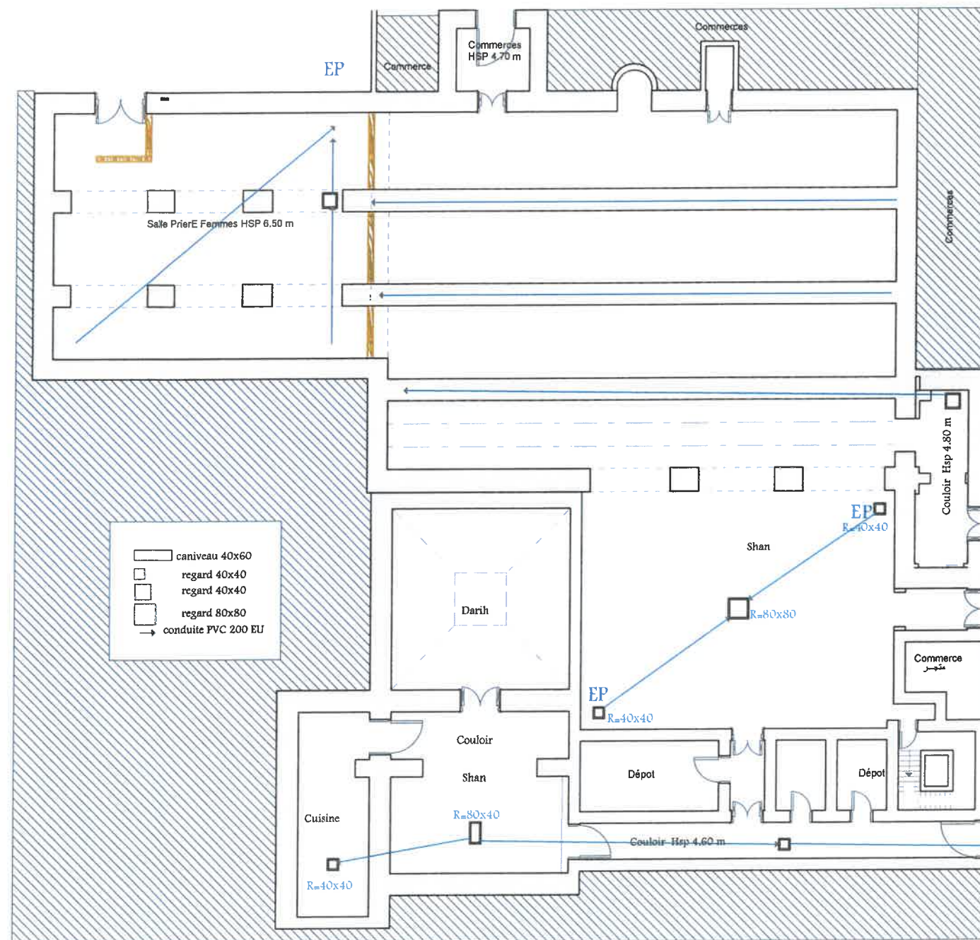
PLAN ASSAINISSEMENT
