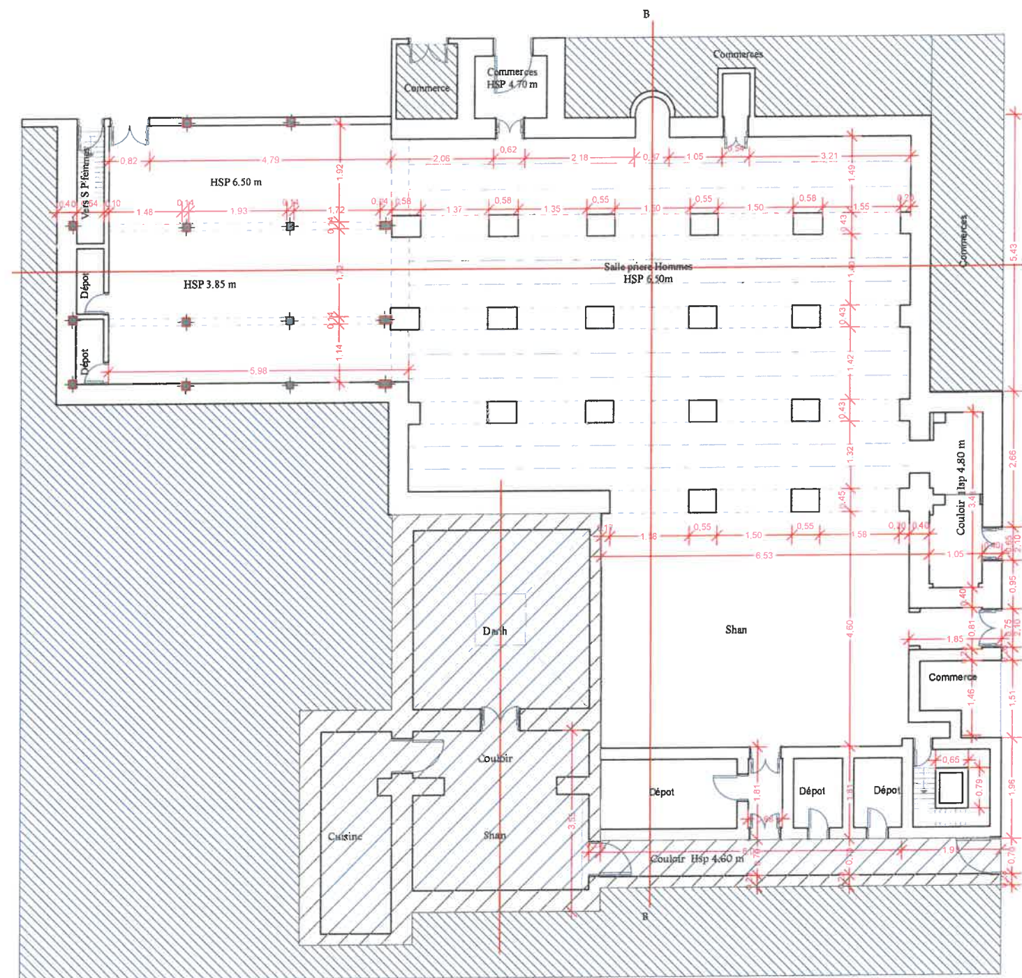
RELEVÉ DE L'EXISTANT REZ DE CHAUSSEE
