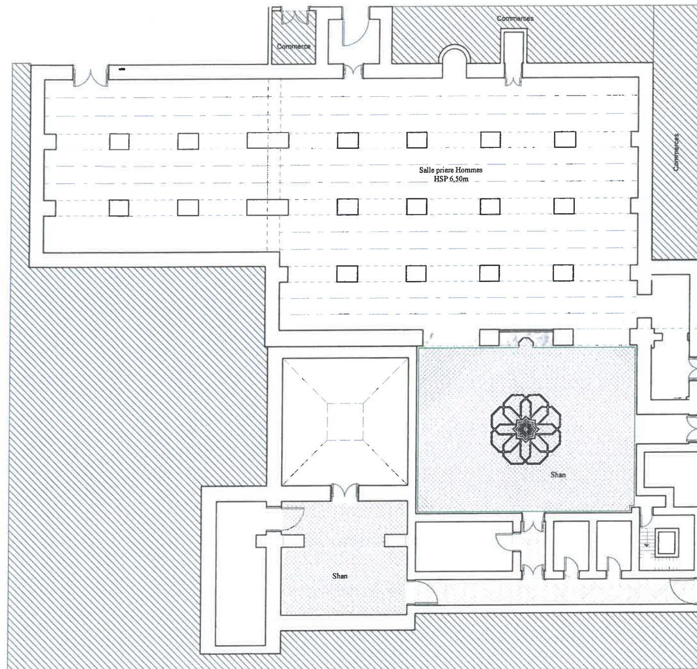
PLAN REVETEMENT
