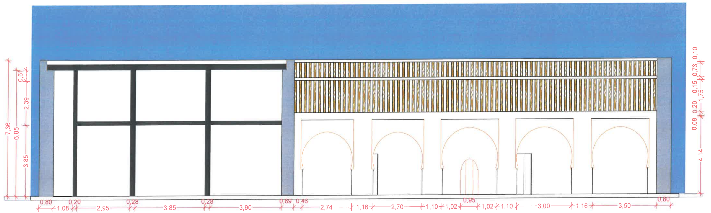
Coupe A A
