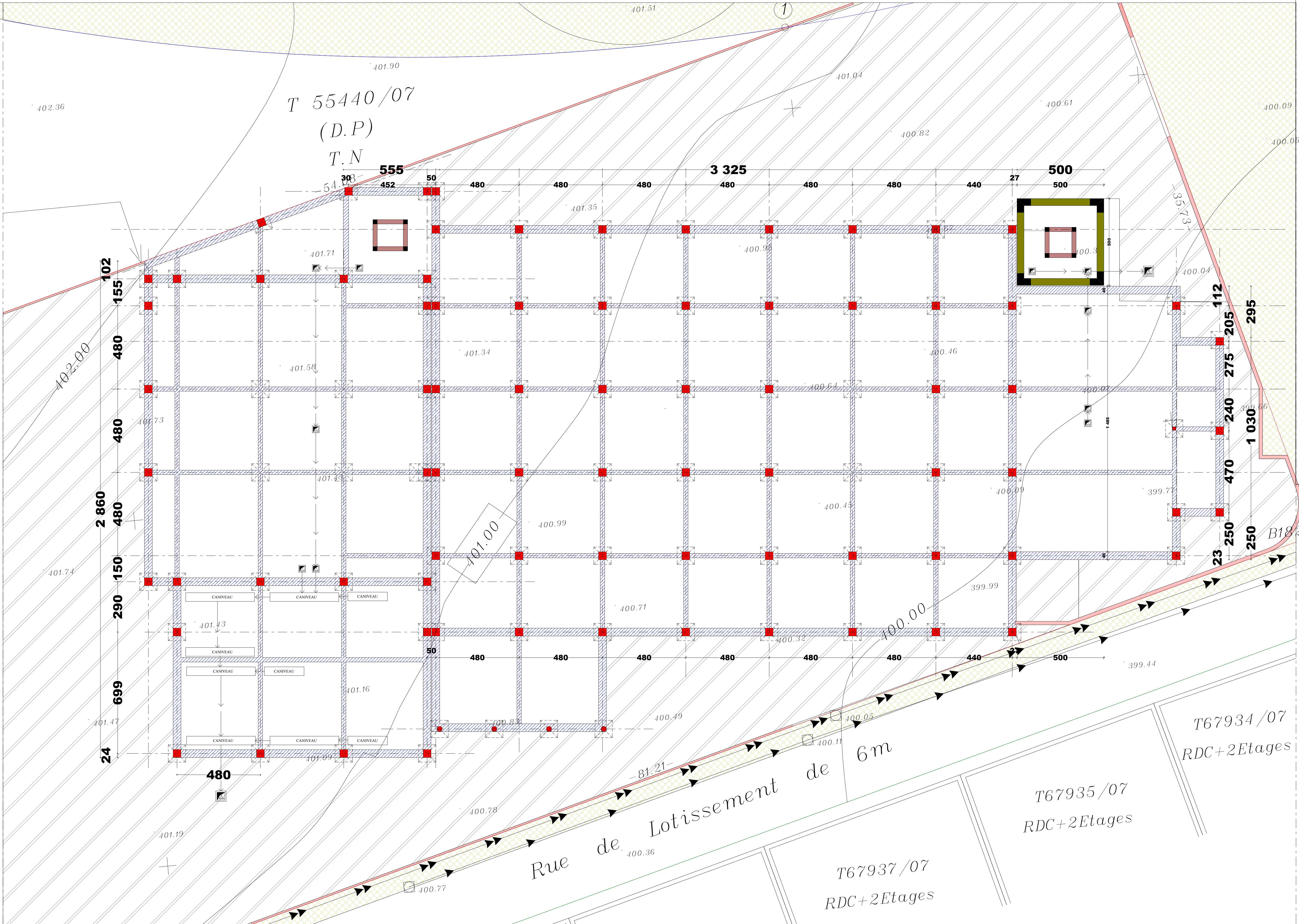
PLAN FONDATION
