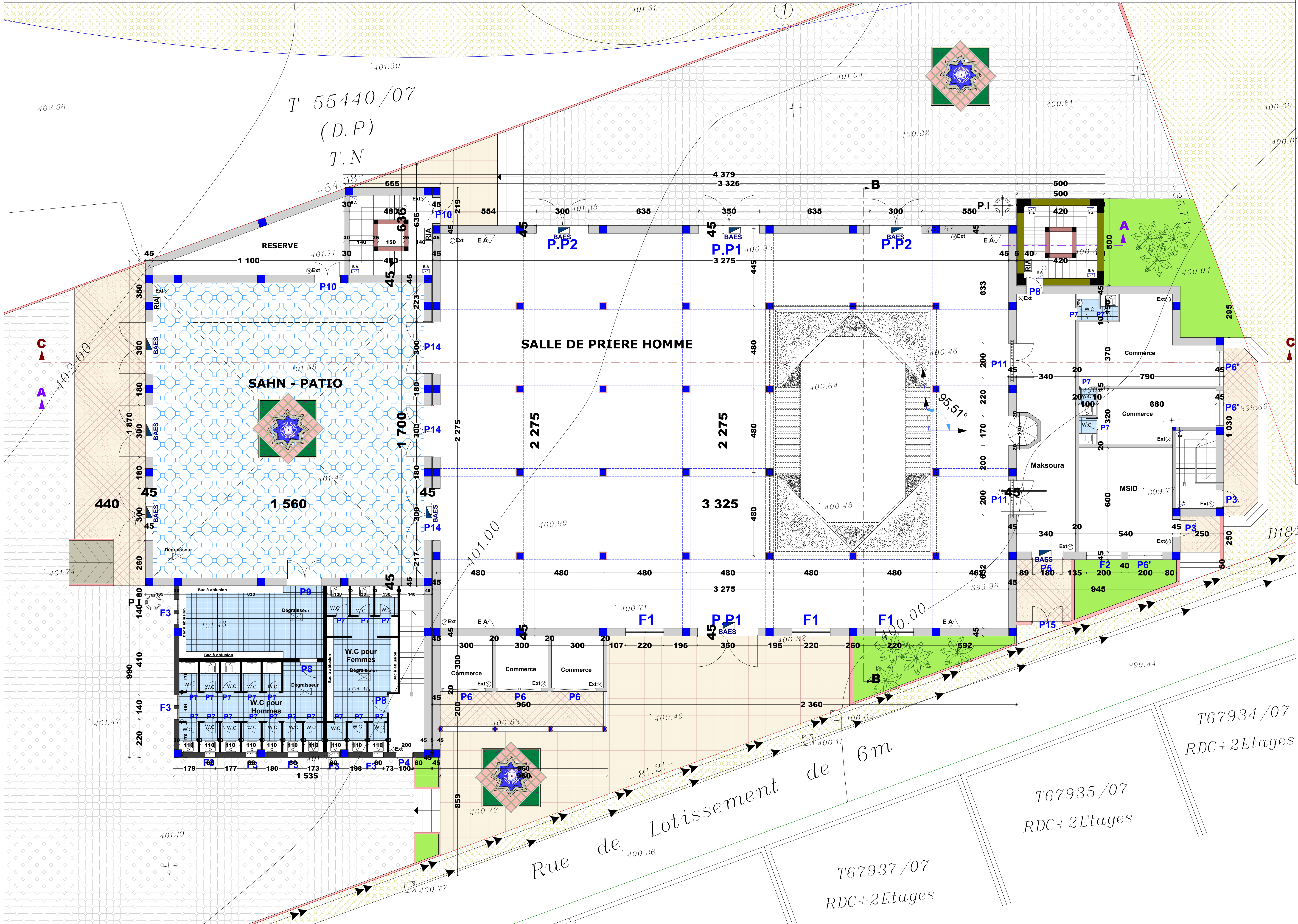
REZ DE CHAUSSEE
